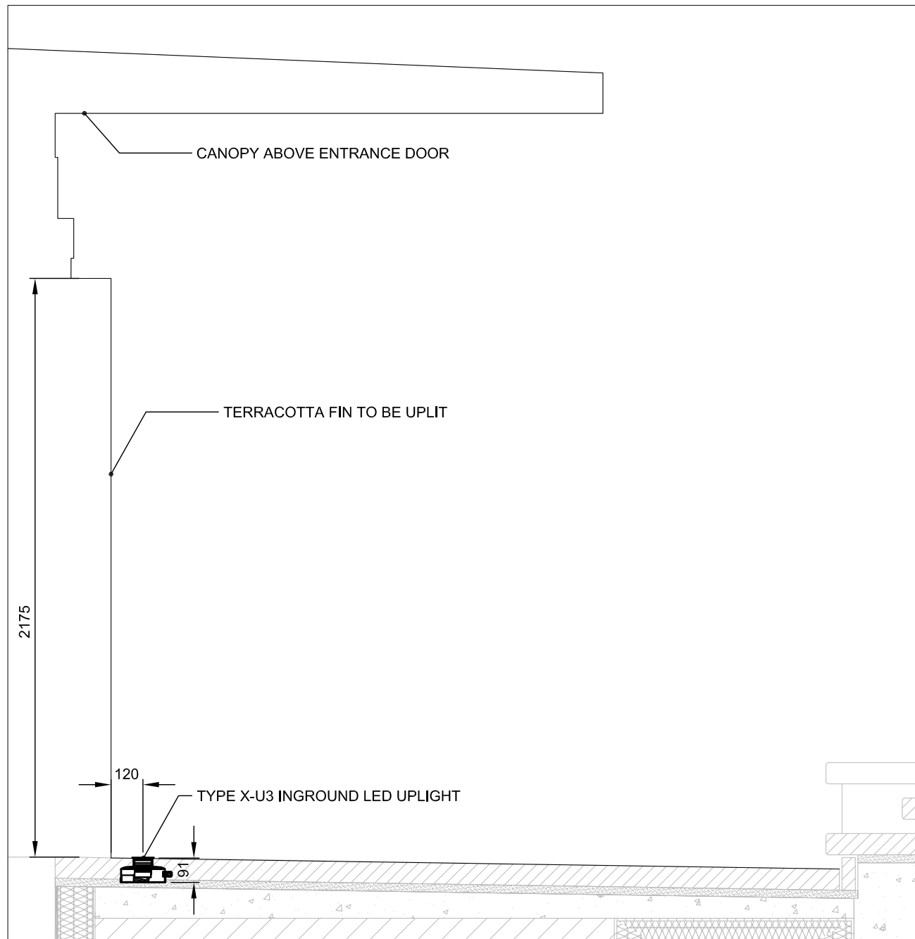
2006 - 1 - TERRACOTTA FIN - SCALE 1:20
