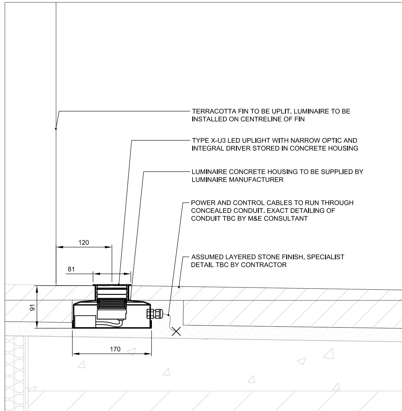
2006 - 2 - TERRACOTTA FIN - SCALE 1:5
